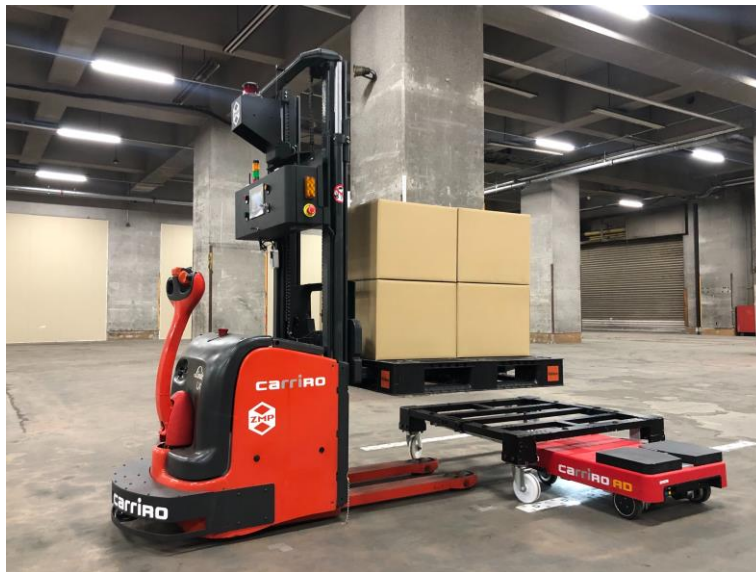
CarriRo®Fork と CarriRo®AD+と連携の様子
